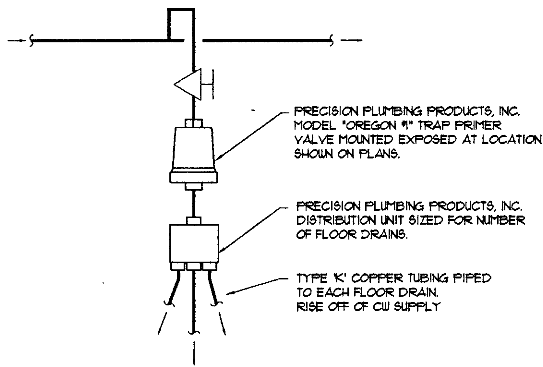
TRAP PRIMER DETAIL
